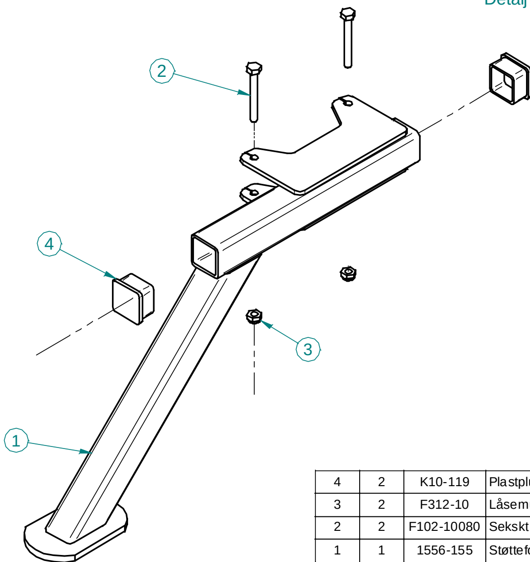
Detalj A
