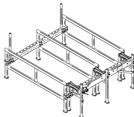
2048-H3 / STOKKESTATIV / 330 kg Hydraulisk / består av: 3 stk seksjoner (2048-020), 1 stk innmattbord med 3 ruller (2048-120), 2 stk lang festeprofil (2048-030), 2 stk staker (2048-034).
