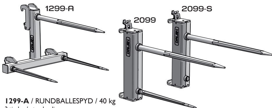
2099 / RUNDBALLESPYD / 31 kg 2 tinder / uten koplingsramme
