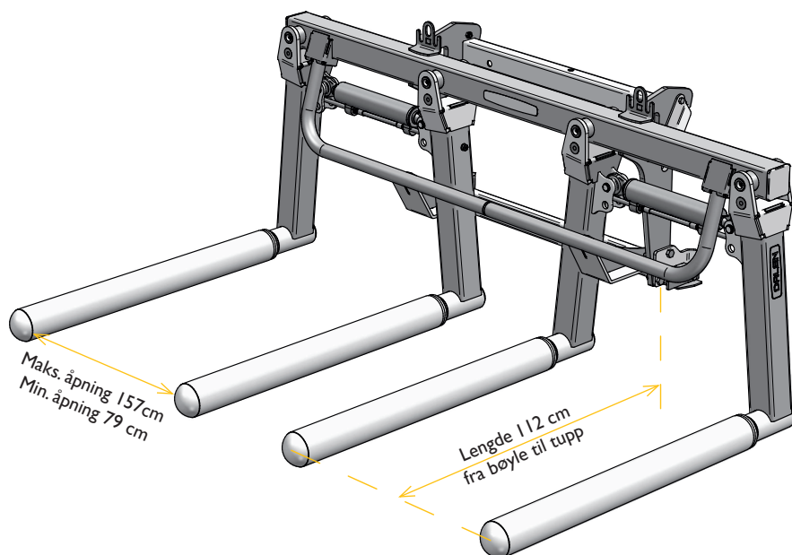
1592 / DOBBEL RUNDBALLELØFTER / 335 kg For standard koplingsramme / uten standard koplingsramme
