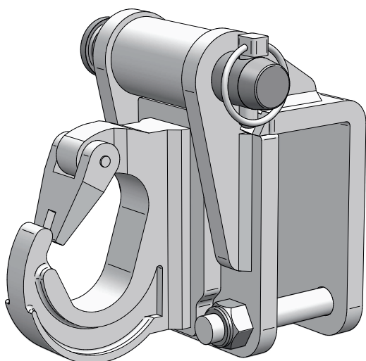
2098 / LØFTEKROK / 8 kg For koplingsramme / uten koplingsramme
