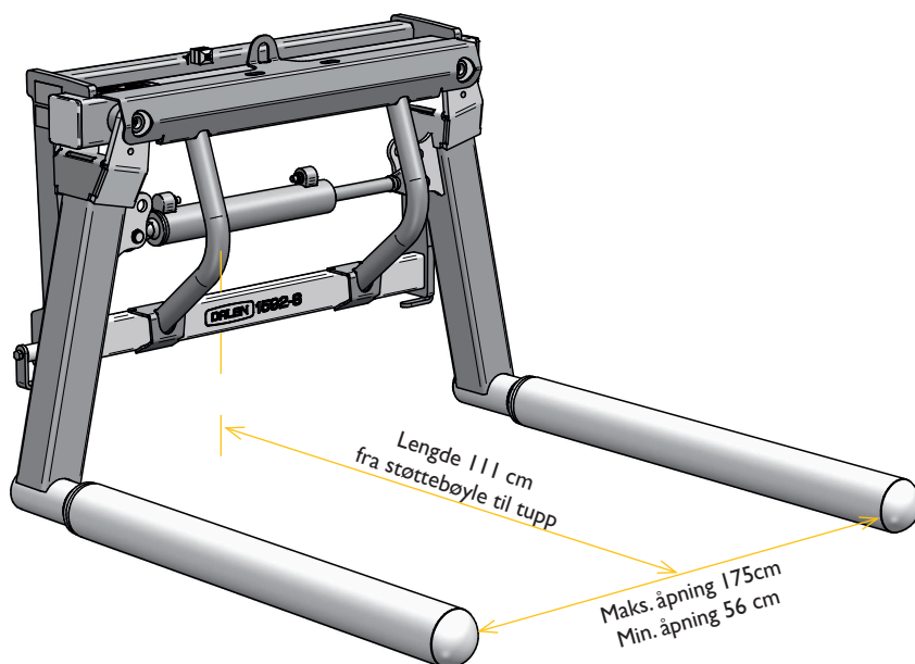
1592-S / RUNDBALLELØFTER / 180 kg For standard koplingsramme / uten standard koplingsramme
