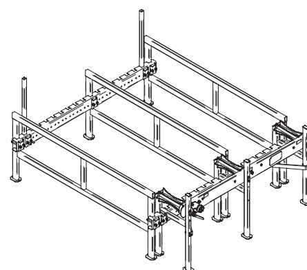
2048-H3 / STOKKESTATIV / 330 kg Hydraulisk / består av: 3 stk seksjoner (2048-020), 1 stk innmattbrett med 3 ruller (2048-120), 2 stk lang festeprofil (2048-030), 2 stk staker (2048-034).
